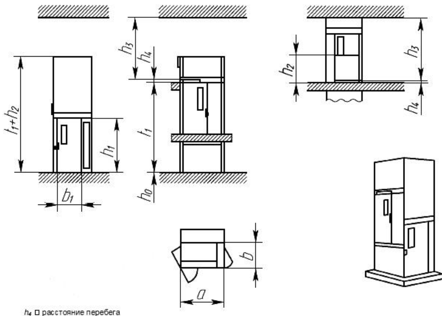
Рисунок 6 - Подъемная платформа с огражденной зоной перемещения
