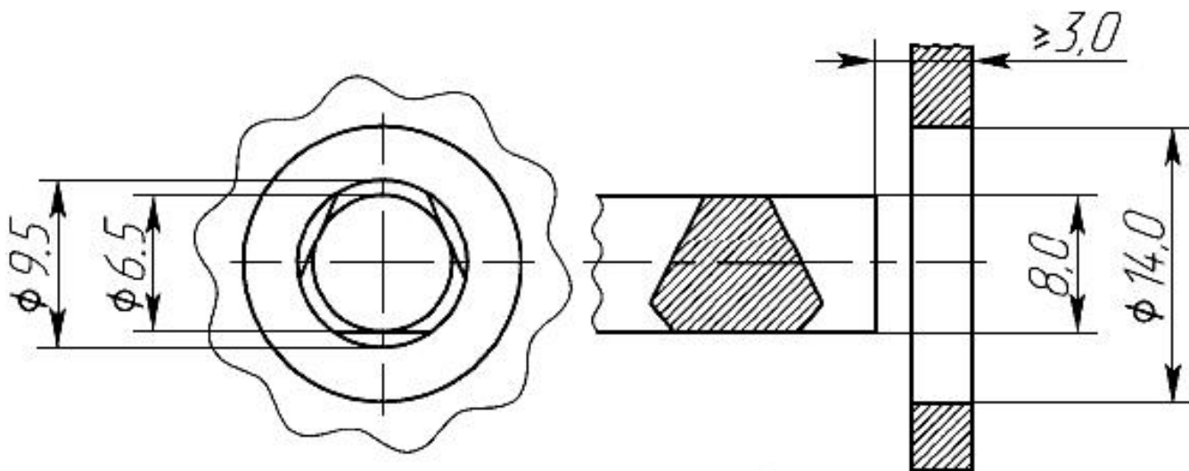
Рисунок 9 - Треугольный ключ для запираения двери по ГОСТ Р 53780
